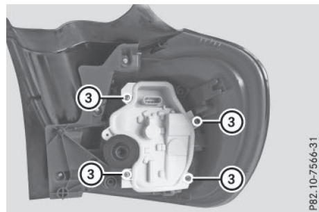
Feux arrière
